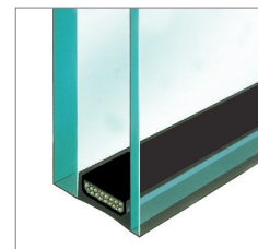
Aufpreis Schallschutzglas Phon 1.1 XN 38 Glasaufbau 10-16-4 mm U_g: 1,1 \text{ (W/m}^2\text{K)}
