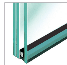
Aufpreis Einbruchhemmendes Glas Safe 1.1 ONE P4A Glasaufbau A3 10-16-4 mm U_g: 1,1 \text{ (W/m}^2\text{K)}
