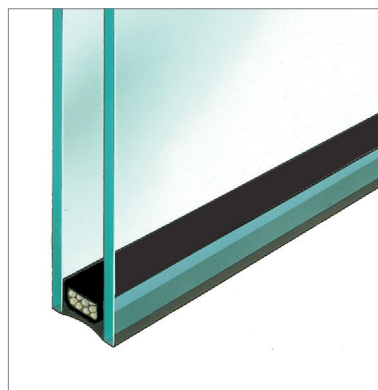
Corona S Wärmeschutzglas Therm 1.1 XN Glasaufbau 4-16-4 mm U_g: 1,1 \text{ (W/m}^2\text{K)}
