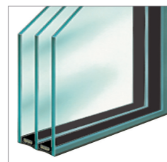
Aufpreis Wärmeschutzglas, 3-fach Therm 0.7 XN Glasaufbau 4-12-4-12-4 mm U_g: 0,7 \text{ (W/m}^2\text{K)}
